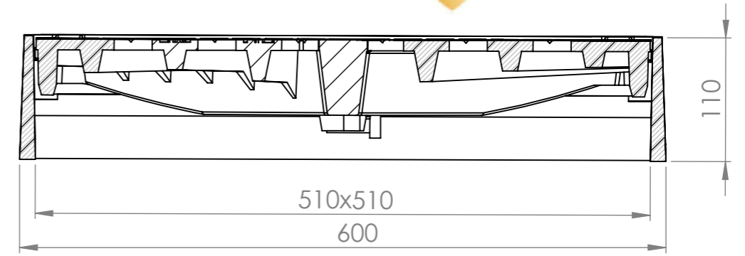
KESIT A-A ÖLÇEK 1 : 5
