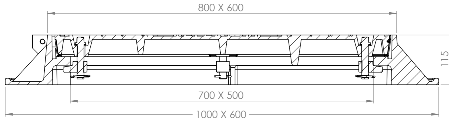
KESIT A-A
