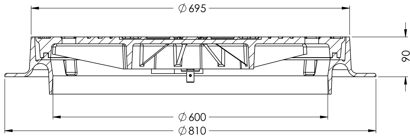
KESIT A-A
